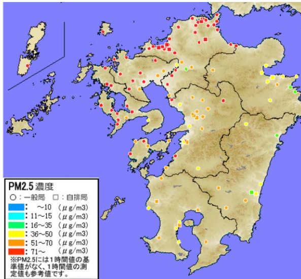
当日12時の九州内PM2.5濃度分布
