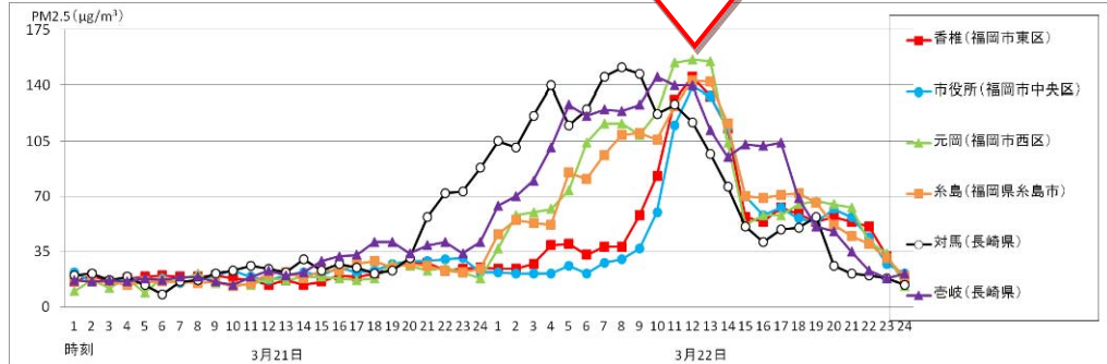
PM2.5濃度推移グラフ
